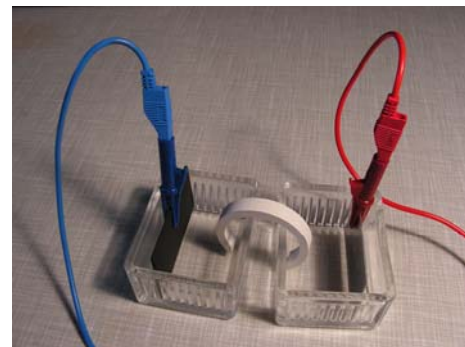
Versuchsbeispiel Halbzellenmethode
