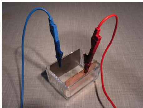
Versuchsbeispiel Elektrolyse
